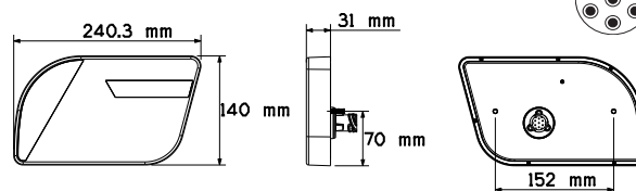
7-polet AMP 1.5 tilslutning
